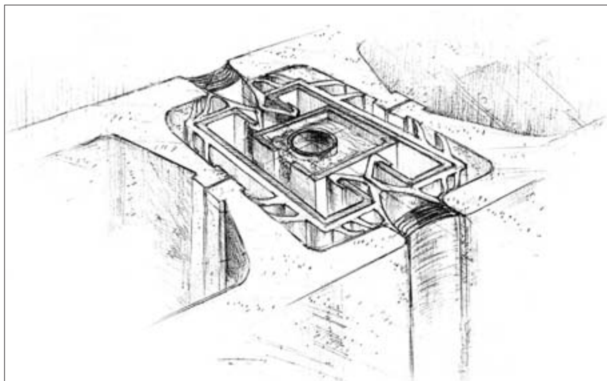
Dettagli di costruzione dei pannelli. Construction details of the panels. Joints between panels SEVES per Renzo Piano
