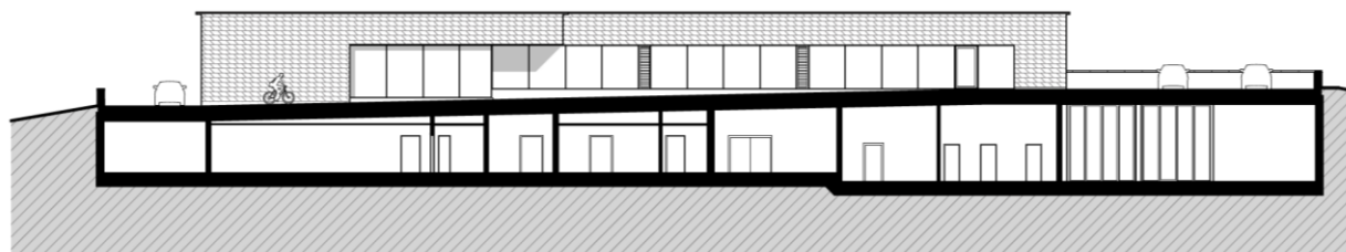
Ansicht Ost Prospetto Est
