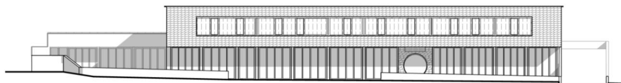
Ansicht West Prospetto Ovest
